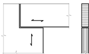
e) Sturz aus BSP eingelegt
