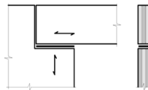
d) ... mit eingelegetem Stahlblech (Auflagerpressung)
